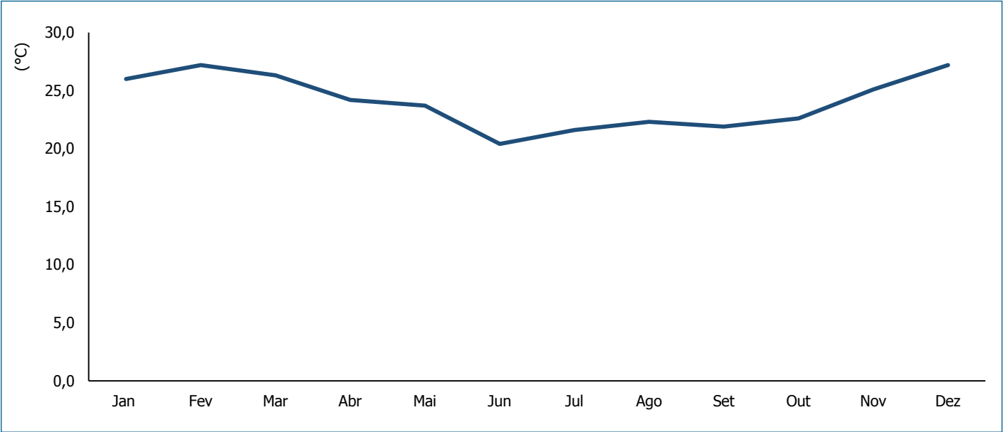
Grafico 1.3.1 Temperatura Média Mensal Registadas, Maputo, 2024/Monthly Average Temperature in Maputo, 2024
