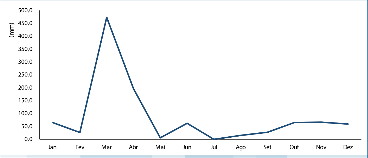
Grafico 1.3.2 Precipitação Mensal Registadas, Maputo, 2024/ Monthly Precipitation in Maputo, 2024
