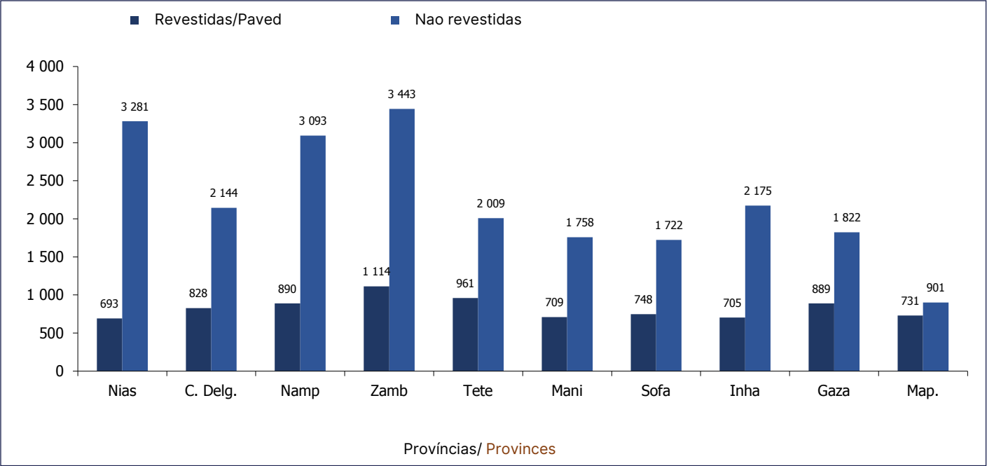
Gráfico 3.9.3.1 Extensão da rede de estradas por tipo de superfície segundo província. Moçambique, 2024/ Road network extension by surface type according to province. Mozambique, 2024
